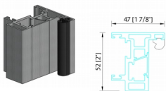
DOOR FRAME PROFILES
